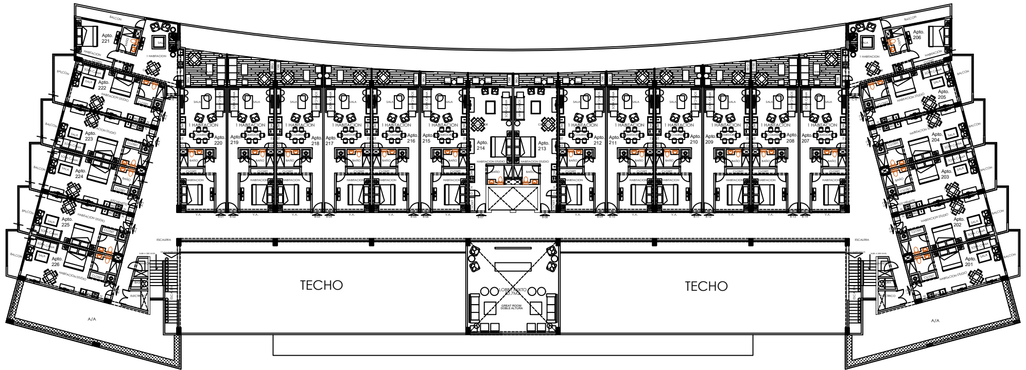
PLANTA ARQUITECTONICA TIPO 2do. al 5to. NIVEL
